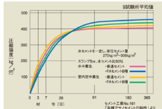
フライアッシュ代替率とマスコンクリートの温度上昇関係試験例
