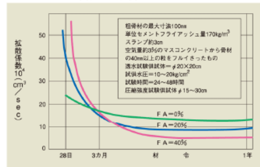
コンクリートの水密性の試験例
