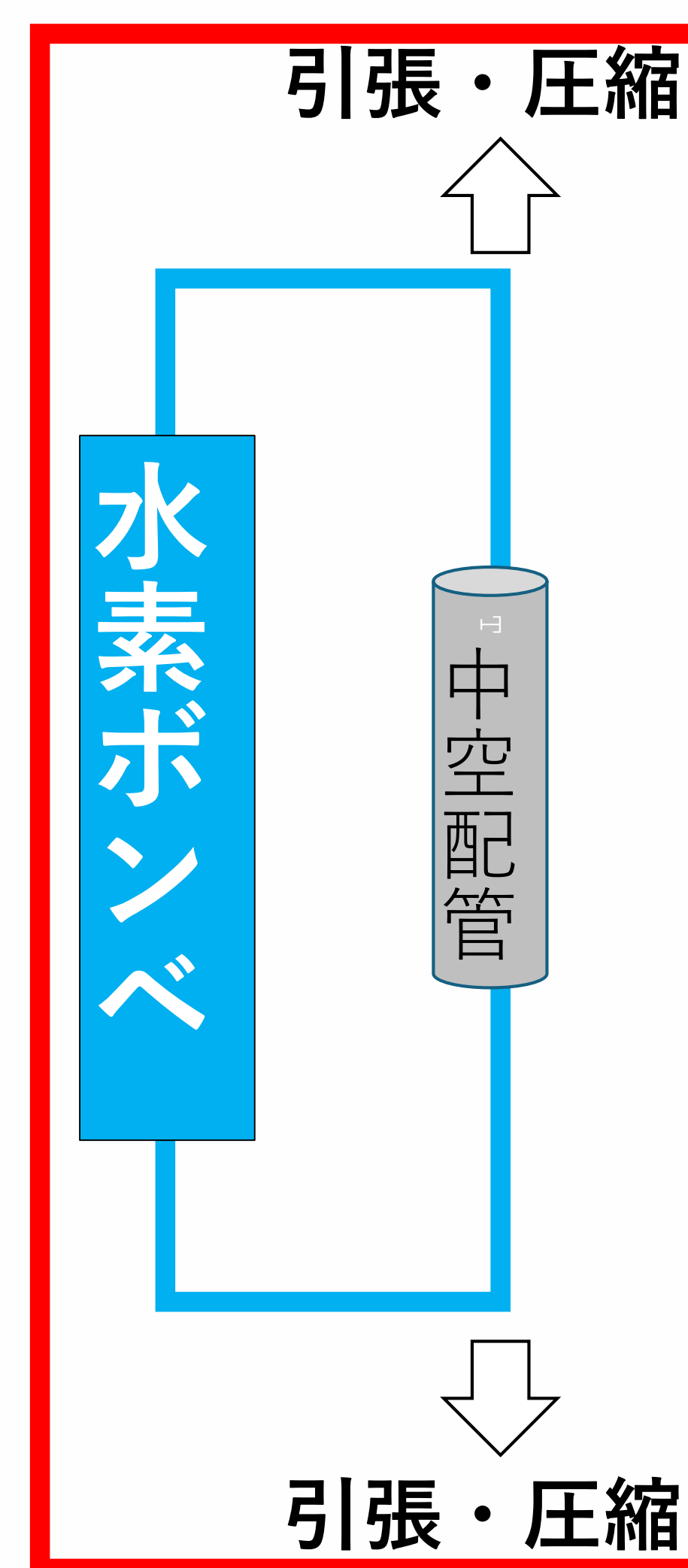
水素環境下疲労試験装置
